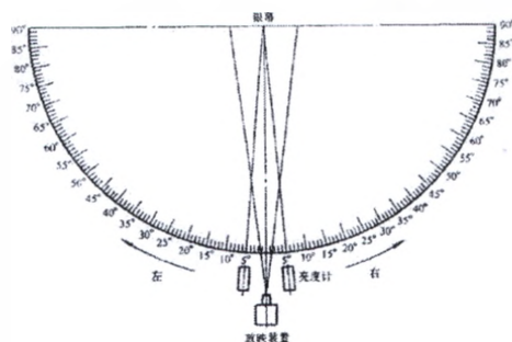
图4 有效散射角测量示意图
