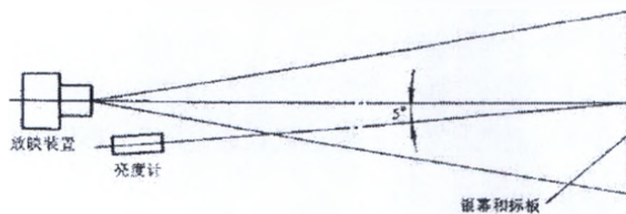
图3 亮度系数测量示意图
