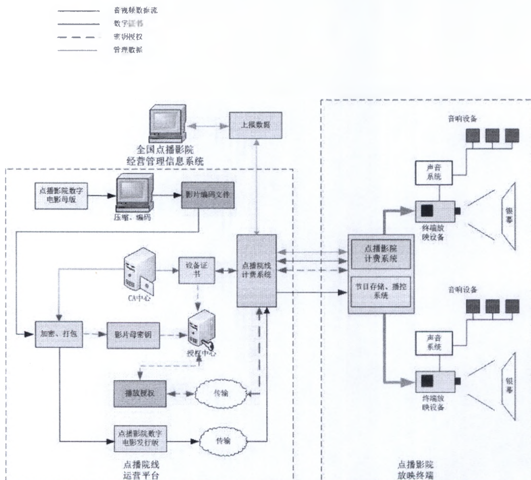
图1 点播影院系统架构示意图
